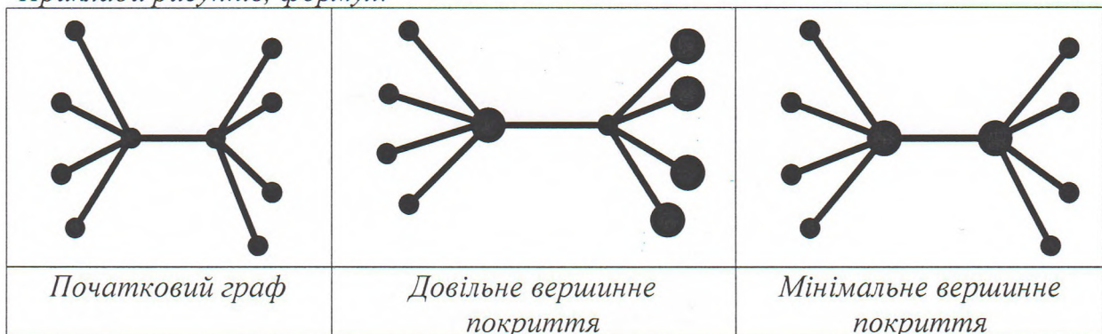
Рис. 1 Вершинне покриття графа
